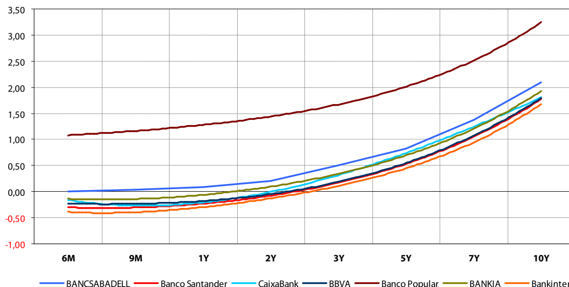
Gráfico 8: Curvas de TIR Emisiones Deuda Simple a 22/02/2017
