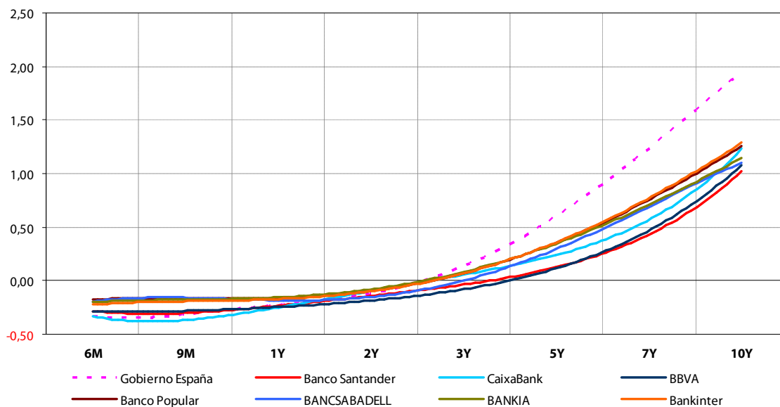
Gráfico 7: Curvas de TIR Cédulas Hipotecarias a 22/02/2017
