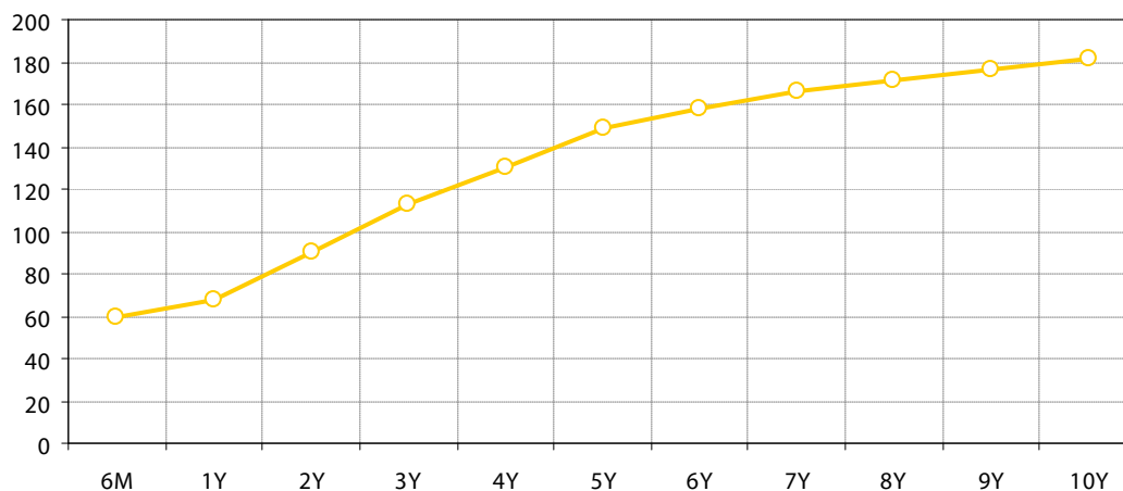
Gráfico 10: Curva de Cotizaciones de CDS de BANCSABADELL para Emisiones de Deuda Senior a 22/02/2017
