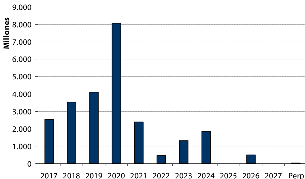
Gráfico 5: Vencimientos de Emisiones de BANCSABADELL (feb-17)
