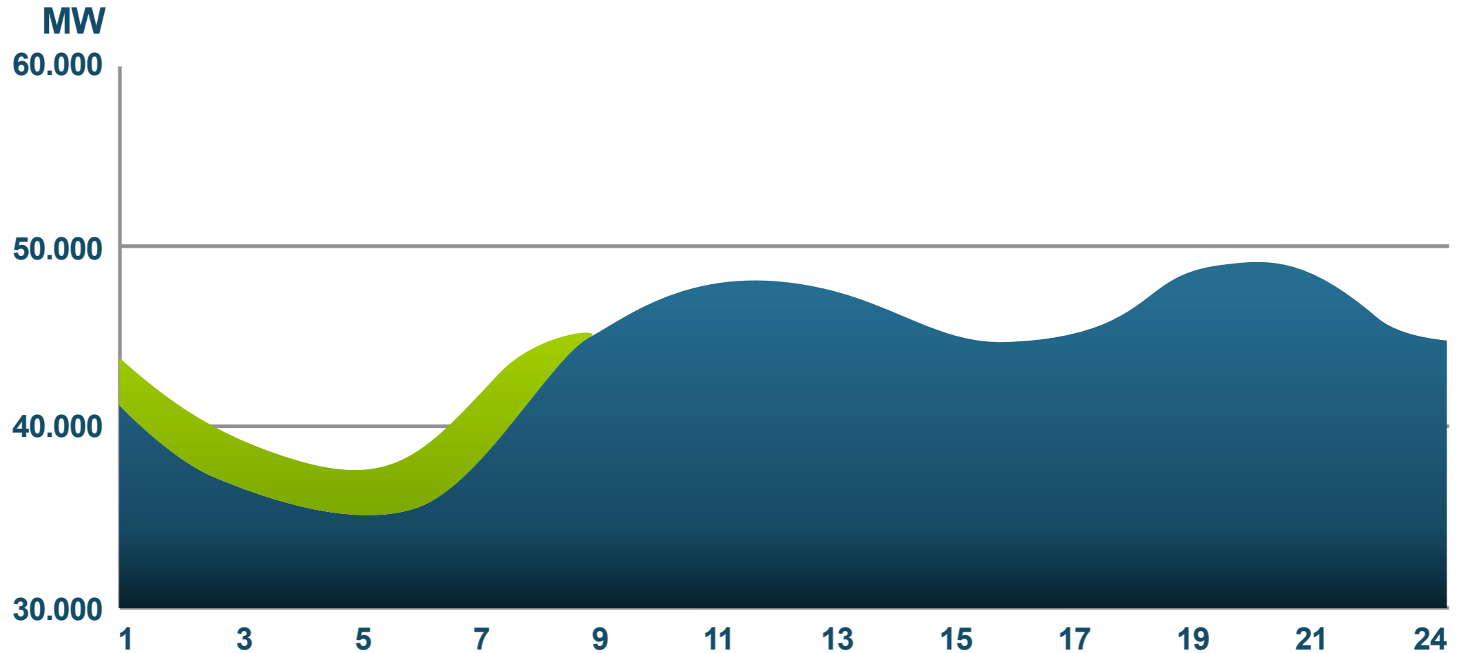
Perfil de demanda para una penetración de un millón de vehículos eléctricos en 2014, recarga simultánea 8 horas (doméstica). Sin gestión inteligente (día tipo invierno)
