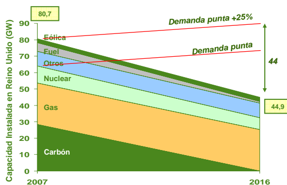
Evolución Capacidad Instalada 2007-2016
