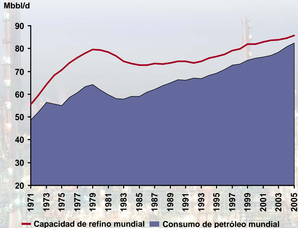
Capacidad de refino frente a consumo de petróleo (2)
